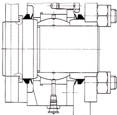
Soporte para perno • V-Seal tipo= VS-0090
