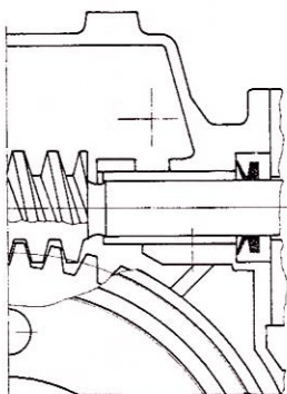
Tornillo helicoidal • V-Seal tipo= VA-0050 Número de vueltas= 1.500/min
