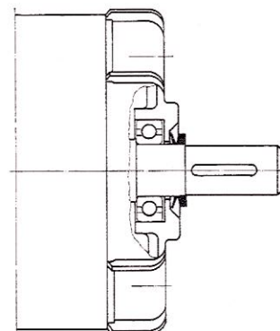
Motor eléctrico • V-Seal tipo= VA-0025 Número de vueltas= 900 a 3.600/min
