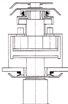
Batidora • V-Seal tipo= VS-0022 e VA-0030 Número de vueltas= 12.000/min
