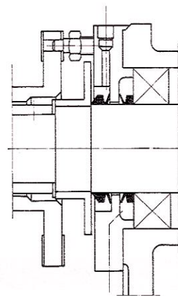
Bomba centrífuga • V-Seal tipo= VS-0050 e VA-0050 • Número de vueltas= 2.000/min
