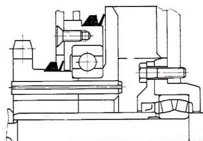
Cilindro vibrador • V-Seal tipo= VS-0110 y VS-0180 Número de vueltas= 30 a 3.000/min
