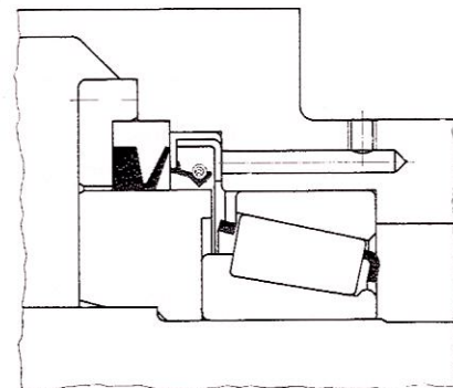
Excavadora • V-Seal tipo= VA-0300 Número de vueltas= 10/min
