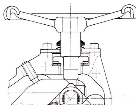
Estanquidad de un tornillo sin-fin • V-Seal tipo= VS-0030 Número de vueltas= 60/min
