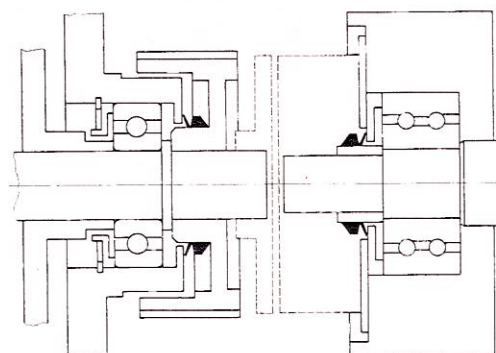
Acoplamiento • V-Seal tipo= VS-0016 y VS-0030 Número de vueltas= 1.300/min
