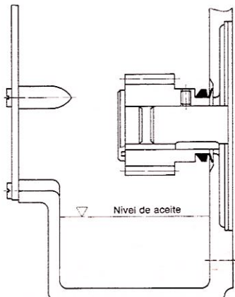
Estanquidad de aceite de una transmisión
