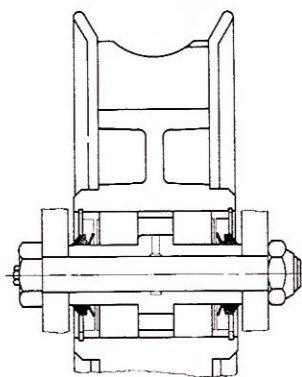
Mecanismo para grúa • V-Seal tipo= VS-0040 Número periférica= 10 m/sec
