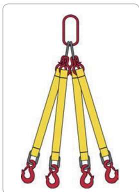
4R Pulpo cuatro ramales Four-leg slings Système 4 brins
